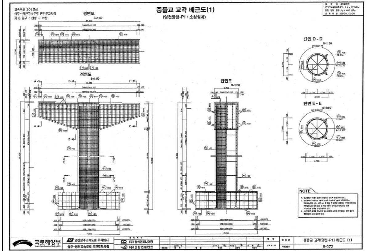
【그림 22.1.13】 교각 배근도
