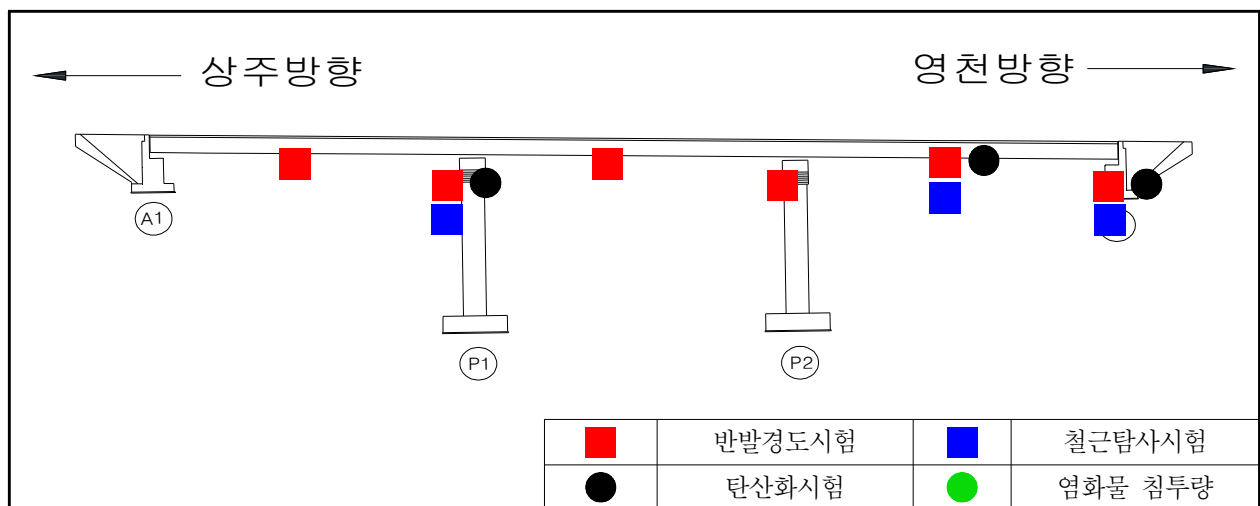
【그림 22.4.2】 영천방향 콘크리트 내구성조사 위치도
