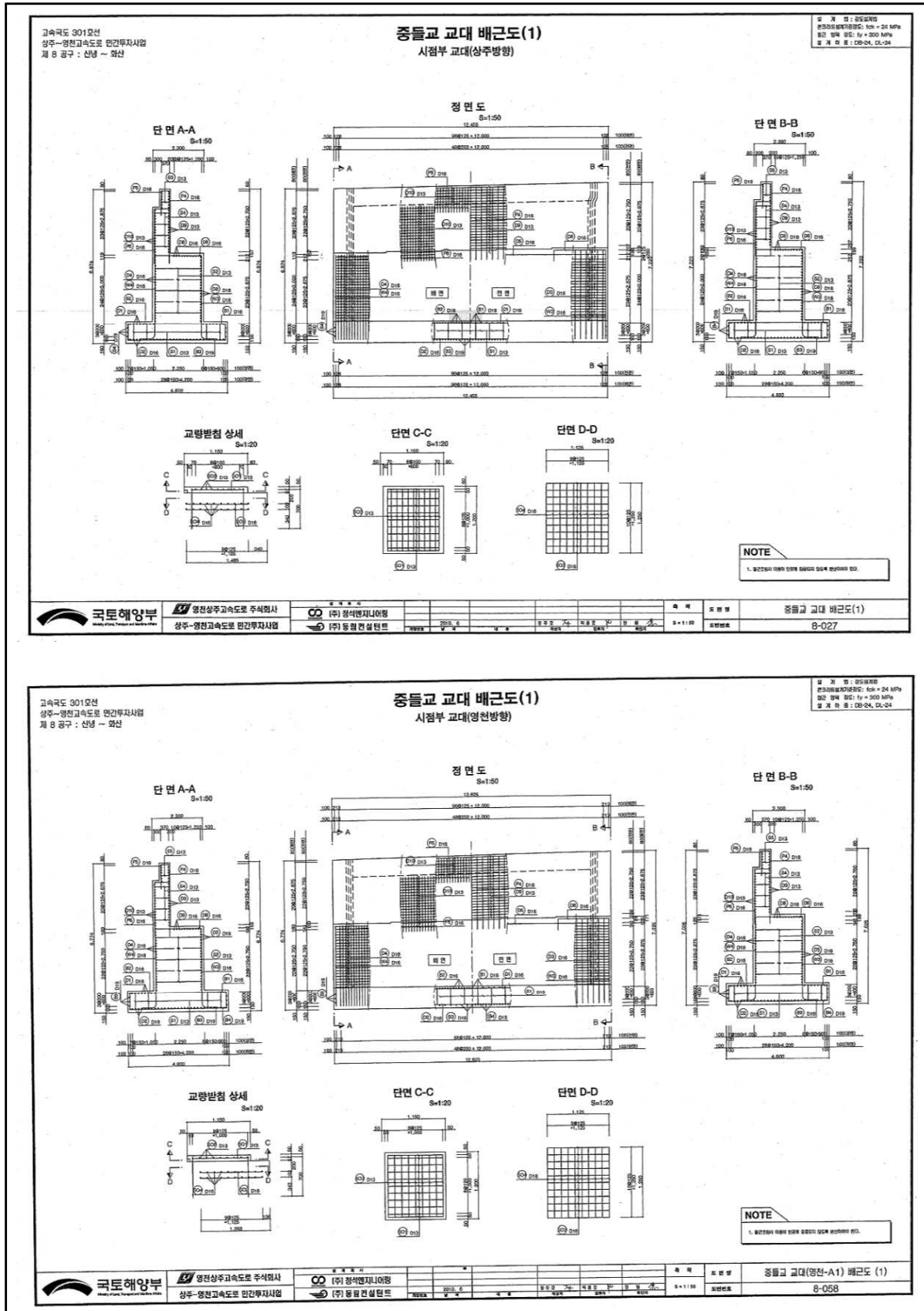
【그림 22.1.12】 교대 배근도
