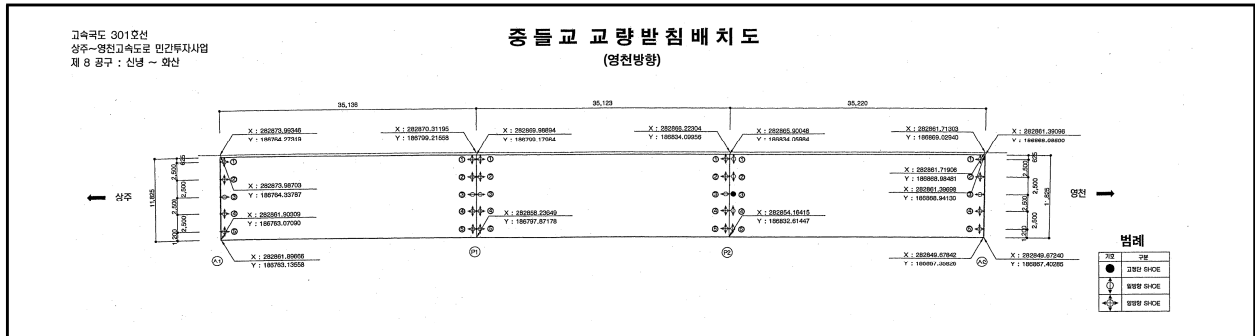
【그림 22.3.3】 교량받침 배치도
