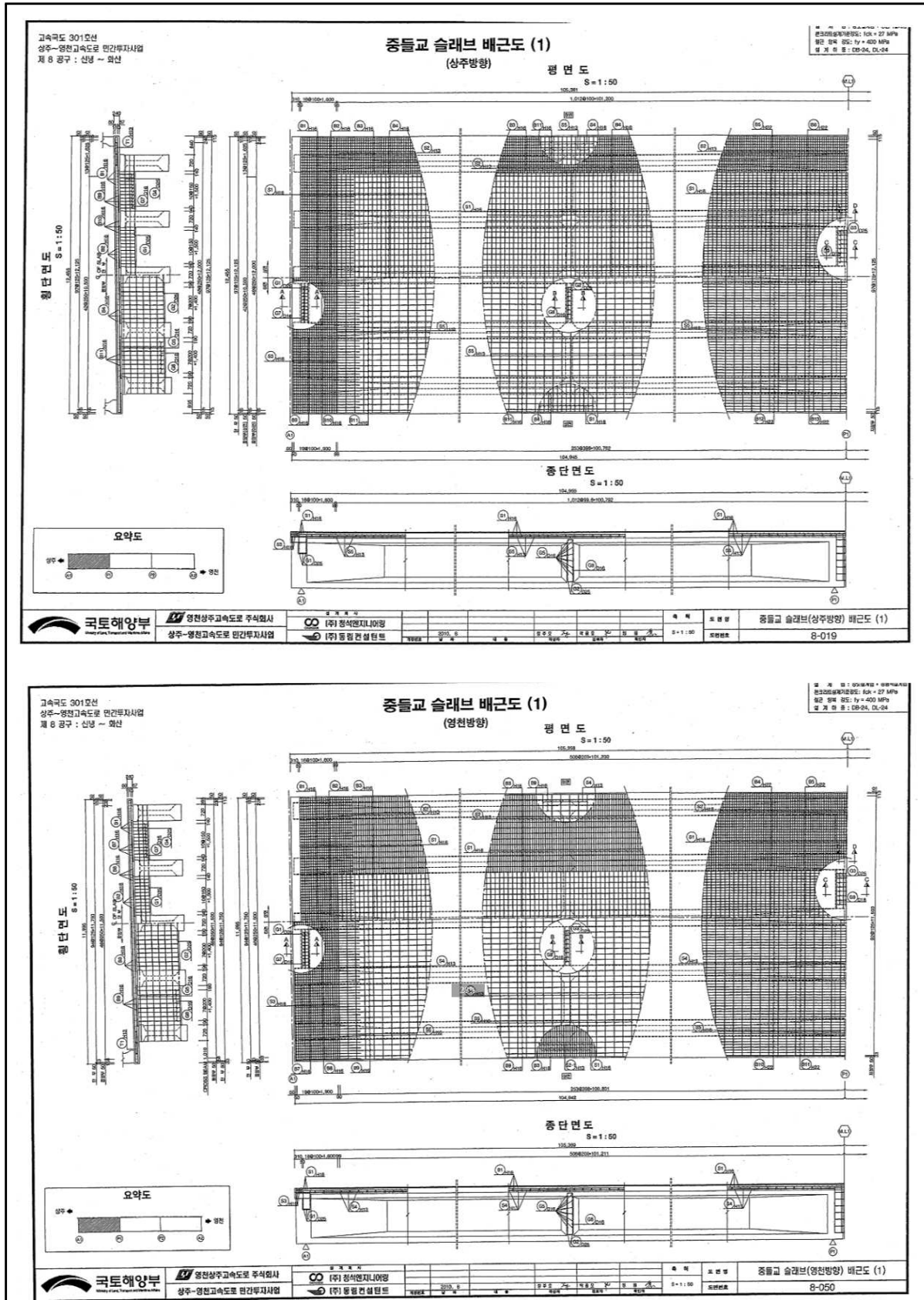
【그림 22.1.11】 바닥판하면 배근도
