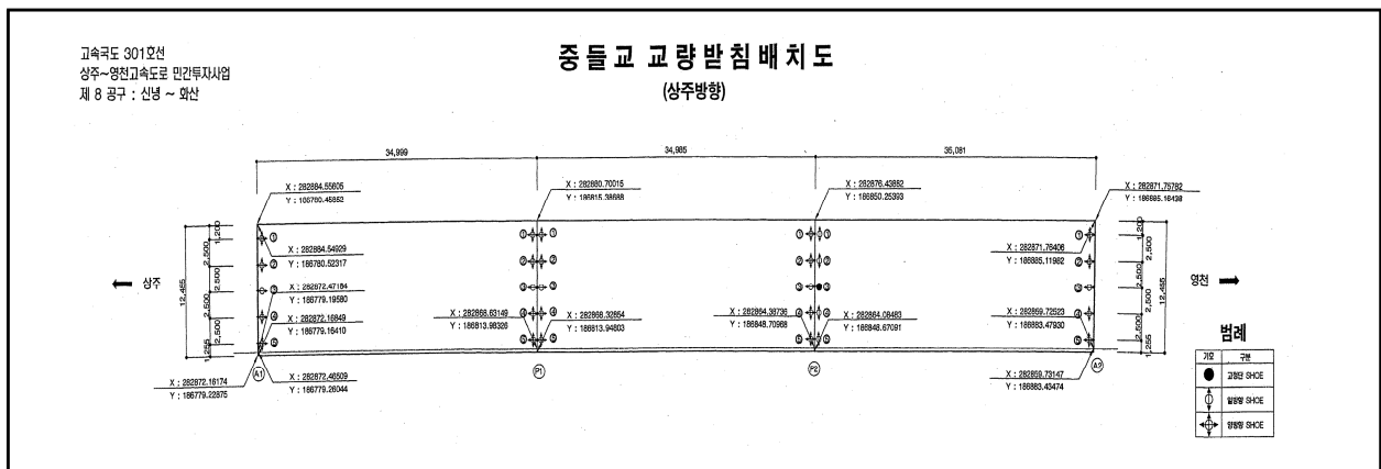
【그림 22.3.1】 교량받침 배치도
