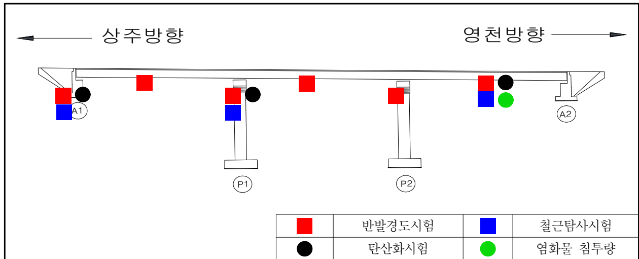
【그림 22.4.1】 상주방향 콘크리트 내구성조사 위치도
