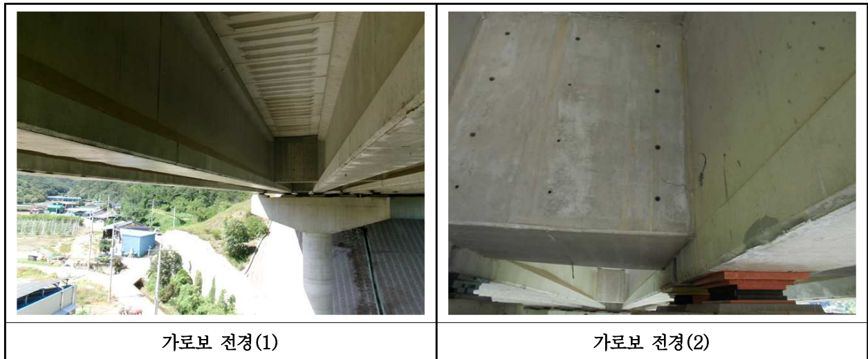
【사진 22.3.31】 가로보 전경
